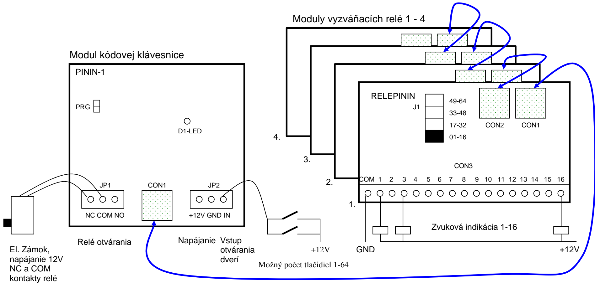
Bloková schéma elektronického kódového zámku PININ-1
